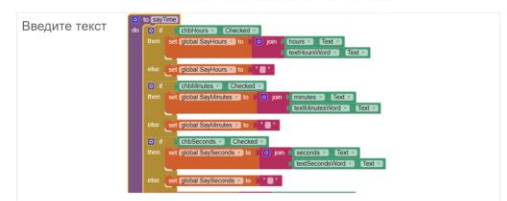
Главная процедура программы
